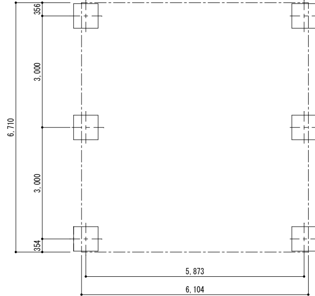
■ 基礎配置図
