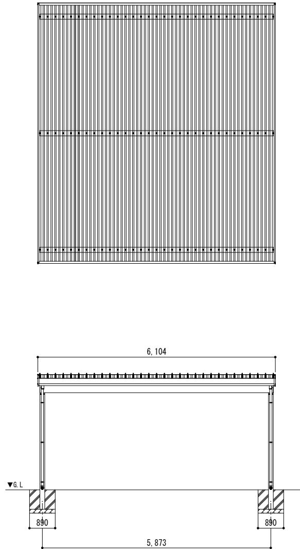
■ 姿図
